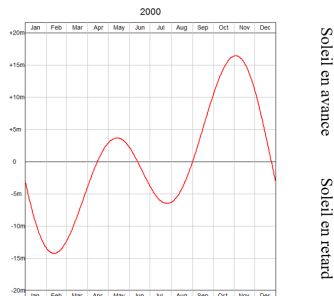
Équation du temps pour l'année 2000 (Théorie VSOP87)
